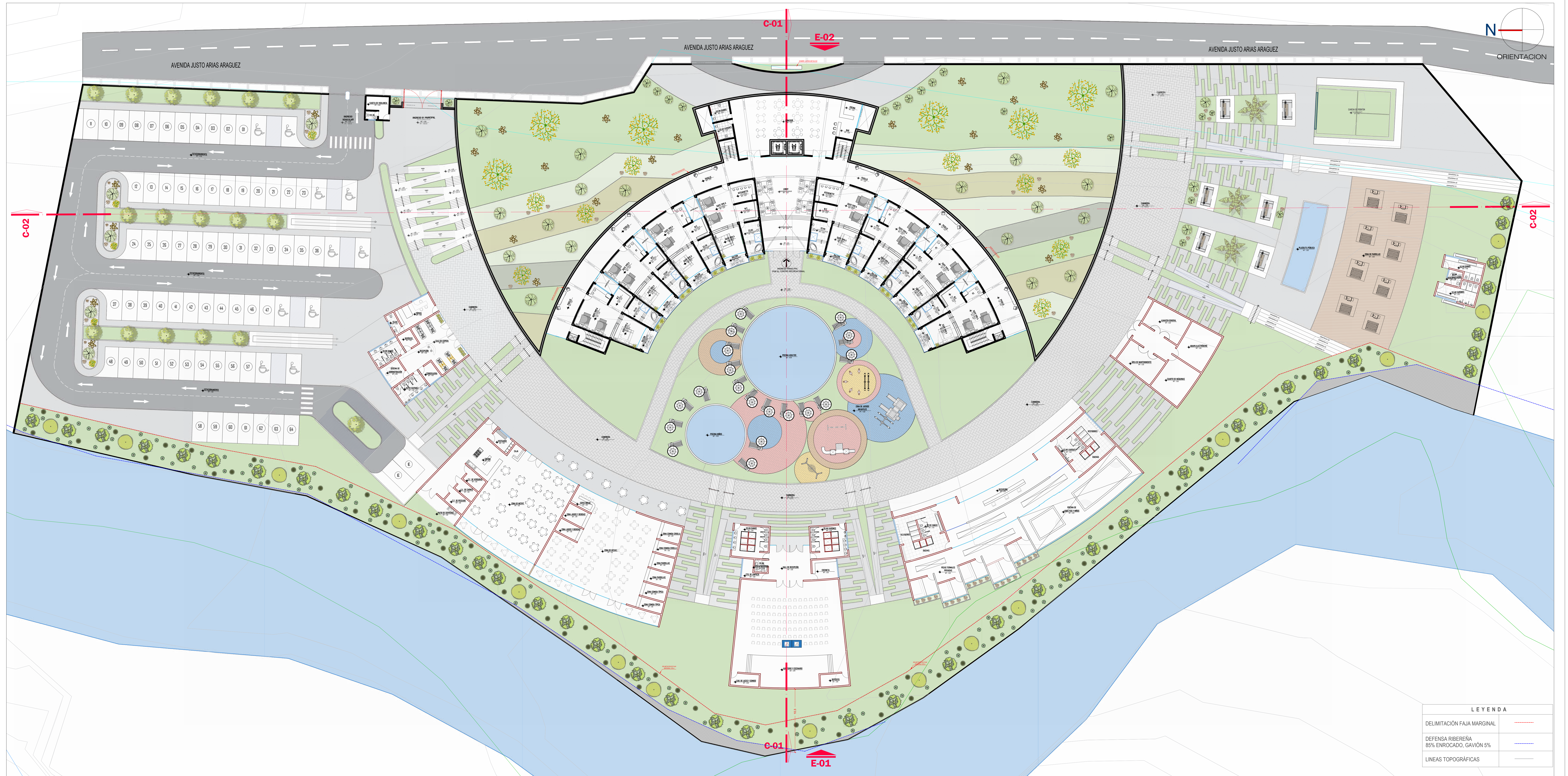
PLANIMETRIA GENERAL ESCALA 1:200
