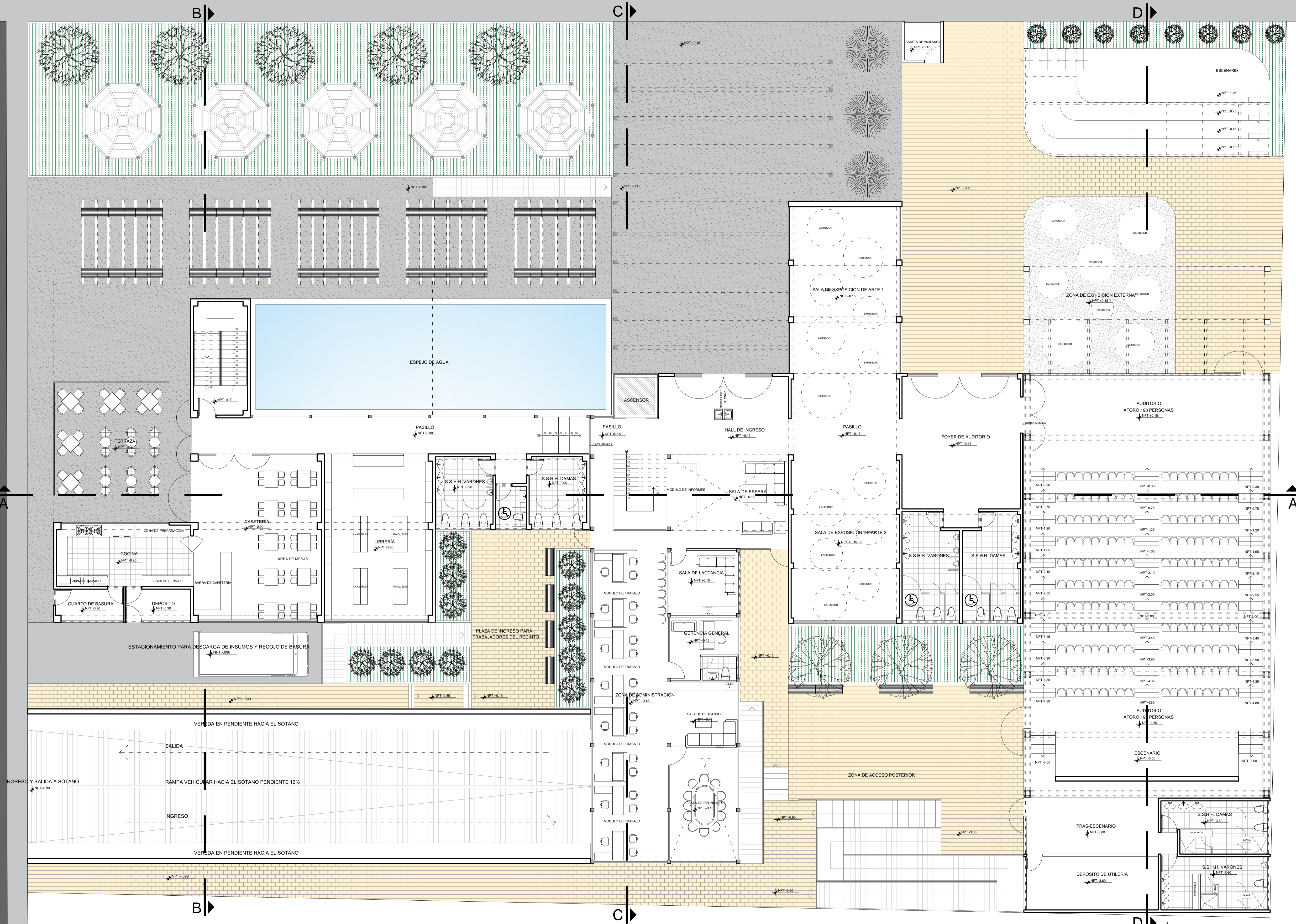
PLANIMETRÍA PRIMER NIVEL ESCALA 1/100
