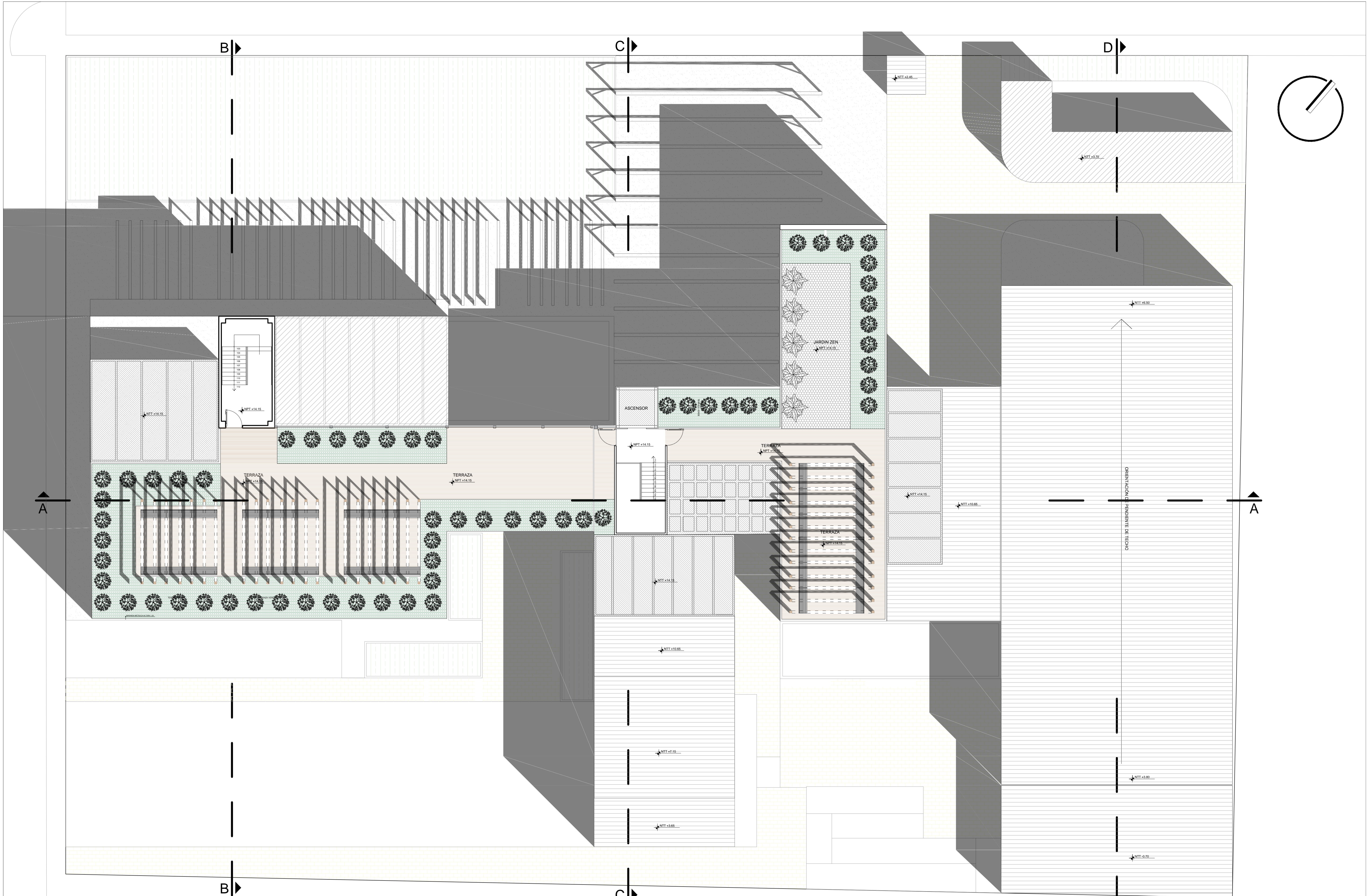
PLANTA DE AZOTEA TIPO PLOT PLAN ESCALA 1/100
