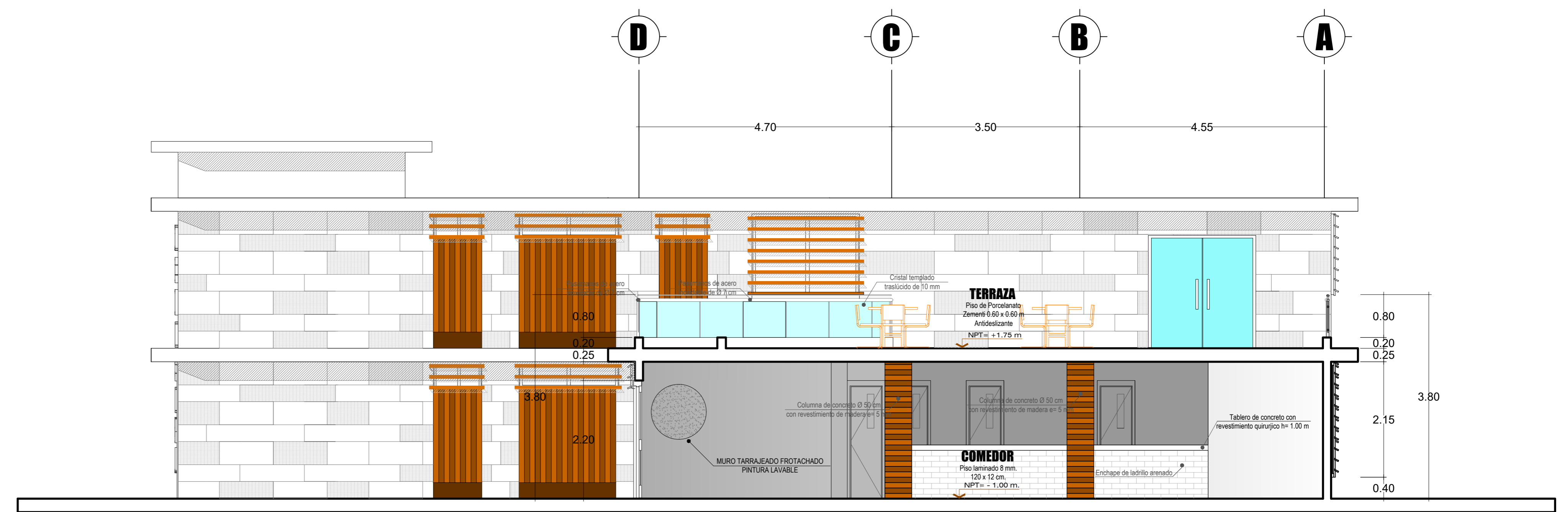
CORTE D - D
