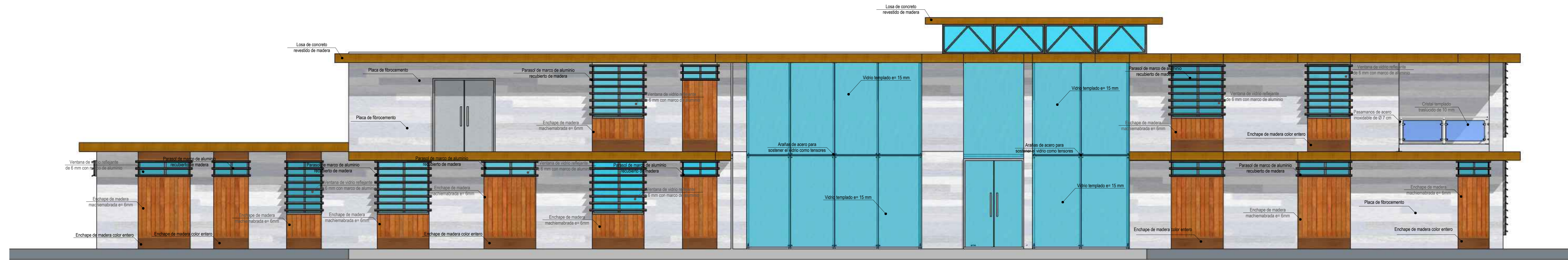
ELEVACIÓN FRONTAL
