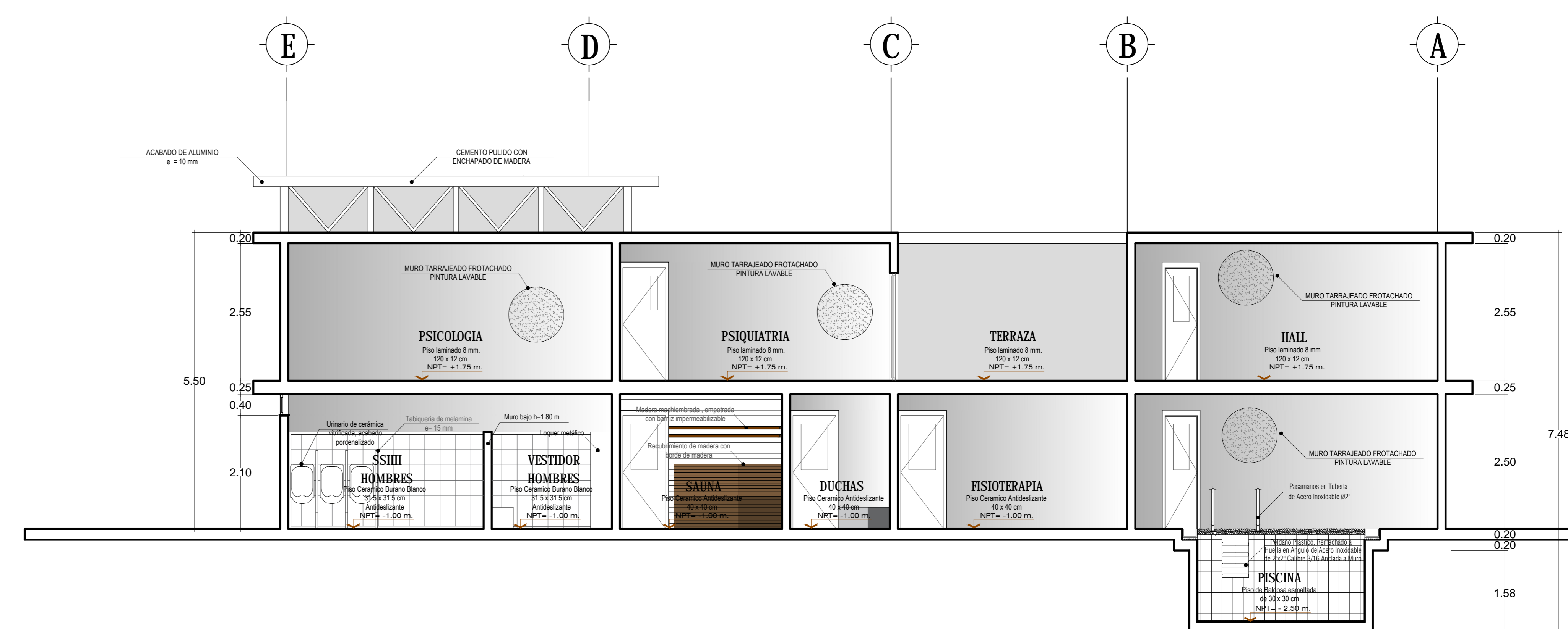
CORTE D - D
