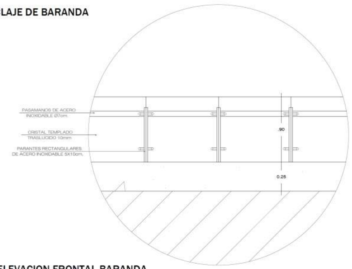
ELEVACION FRONTAL BARANDA ESC: 1/10
