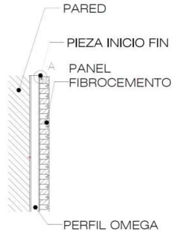
VISTA LATERAL CLIP SUJECION ESC: 1/10
