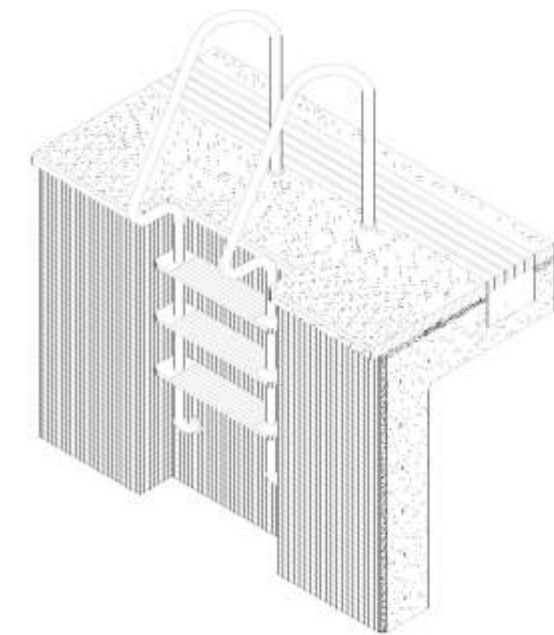
ISÓMETRICO DE BARANDA ESC: 1/10
