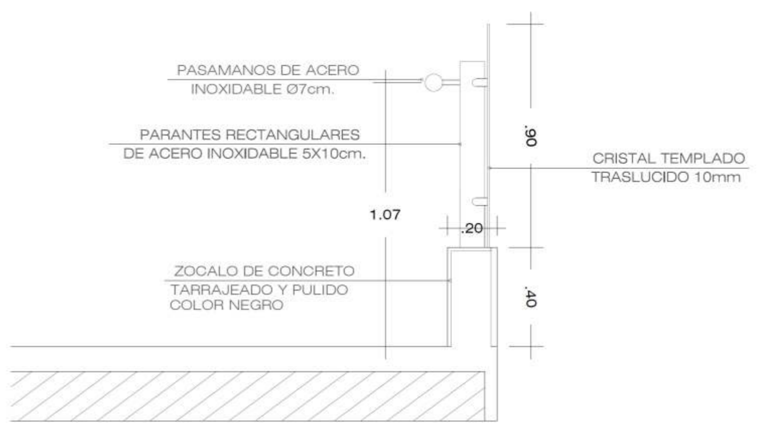
CORTE - ANCLAJE DE BARANDA ESC: 1/5
