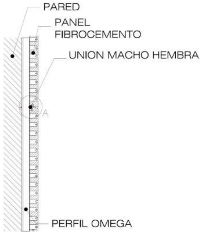
VISTA LATERAL INICIO / FIN ESC: 1/10
