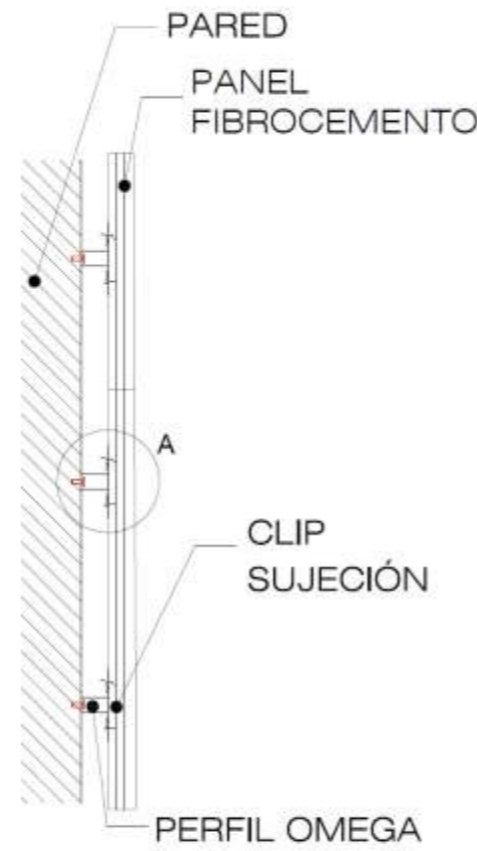
CORTE - ANCLAJE DE PLACA DE FIBROCEMENTO ESC: 1/10
