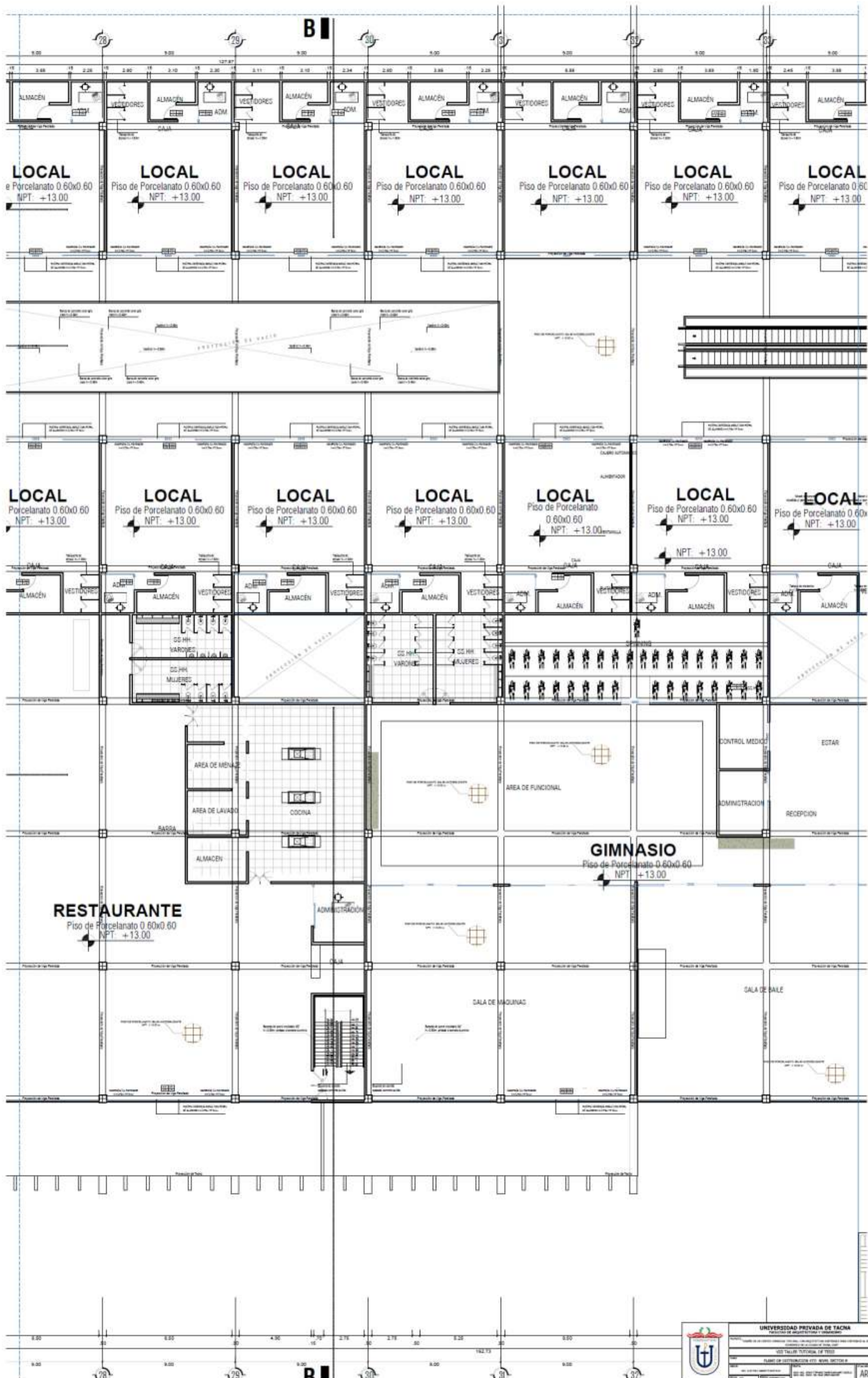
PLANO CLASE PROYECTO
