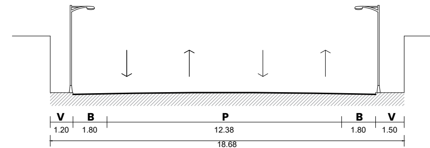
SECCIÓN VIAL 3 - 3' AV. MIRAFLORES ESC: 1/200
