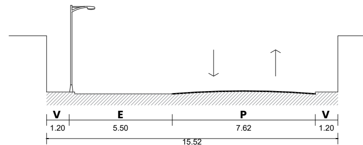
SECCIÓN VIAL 1 - 1' CAL SAN HILARIÓN ESC: 1/200
