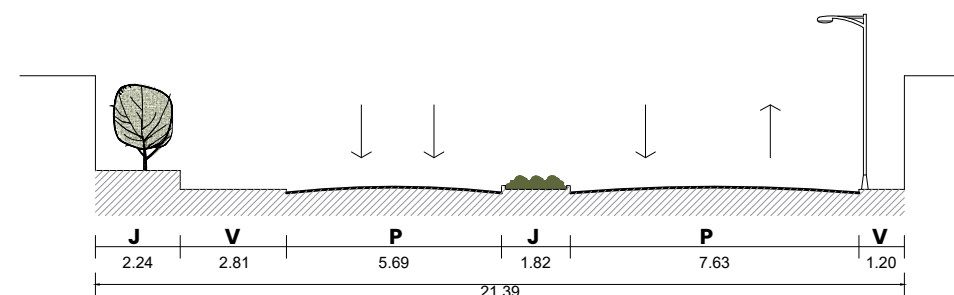
SECCIÓN VIAL 2 - 2' CAL SAN HILARIÓN ESC: 1/200
