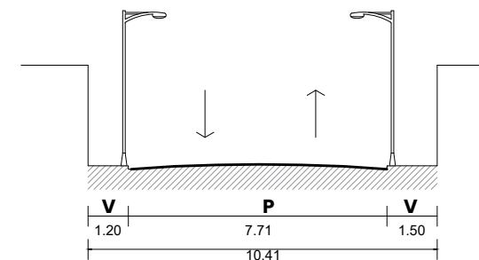
SECCIÓN VIAL 4 - 4' VÍA PROYECTADA ESC: 1/200
