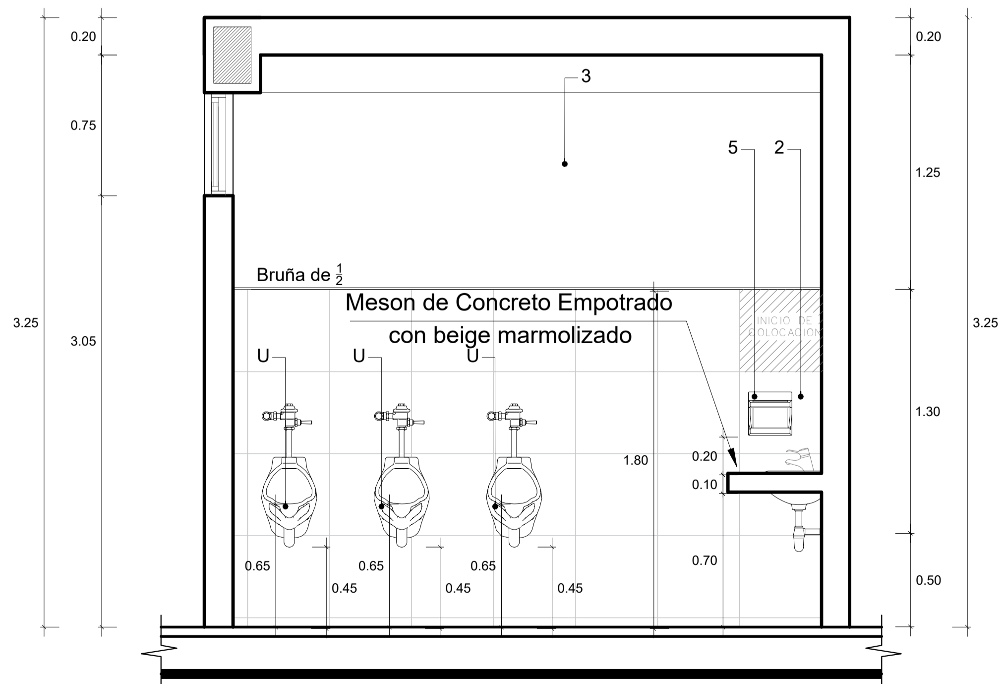
CORTE B - B SS.HH. DE NIÑOS TIPO A
