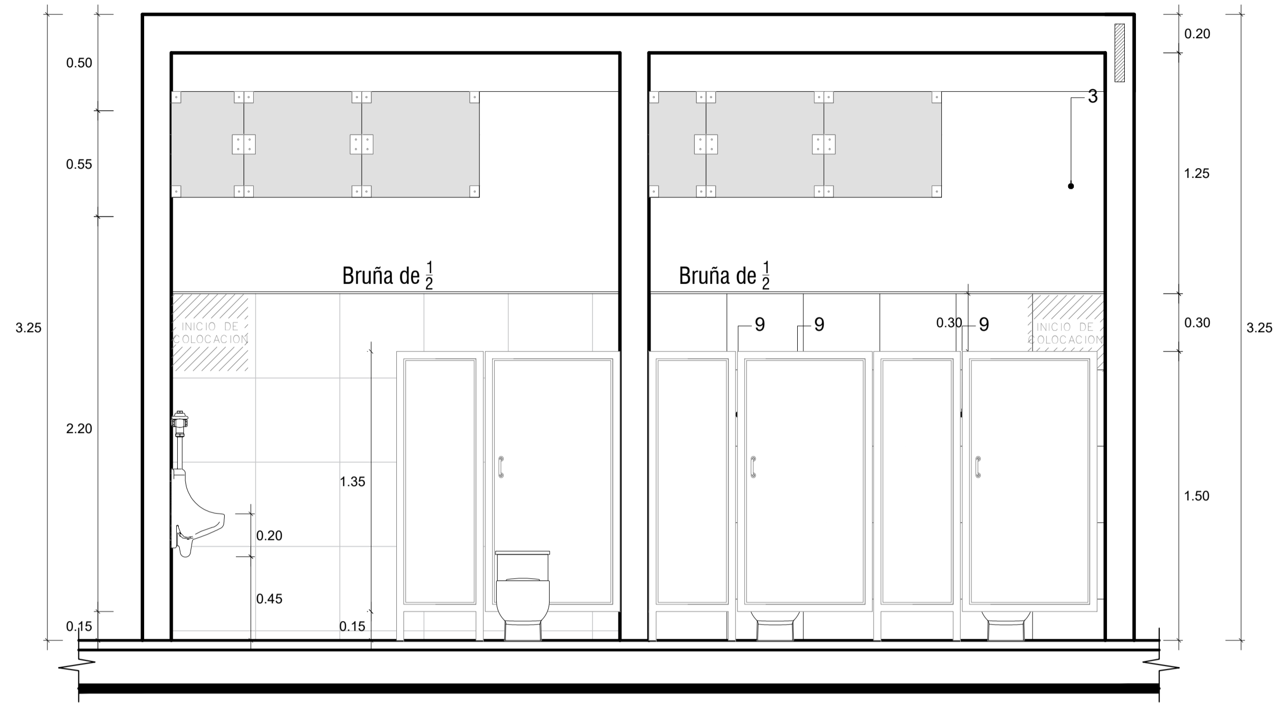
CORTE A - A SS.HH. DE NIÑOS TIPO B
